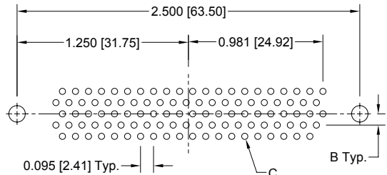
ODD104 MALE
